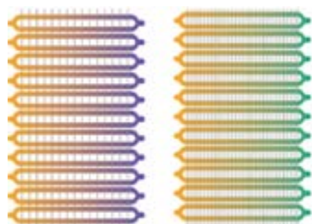
Обычная VRF-система
