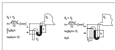
РАСЧЕТ СИФОНОВ СТОКА КОНДЕНСАТА
