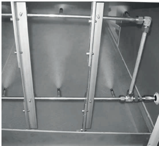
Система форсунок
