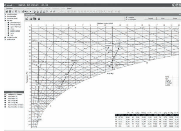
h-x диаграмма
