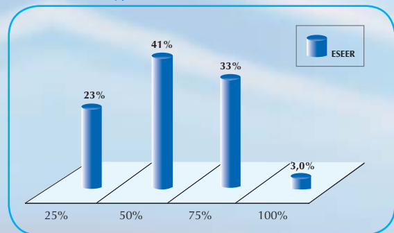
Распределение количества полезной мощности при различных нагрузках согласно показателю ESEER
